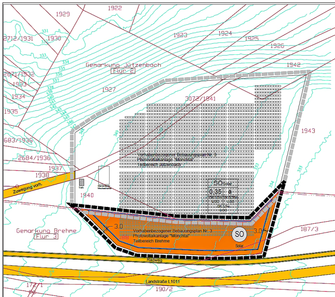
Übersicht Geltungsbereich Vorhabenbezogener Bebauungsplanes Nr. 3, Photovoltaikanlage „Mönchtal“ - Teilbereich Brehme und 2. Änderung des Flächennutzungsplanes der Gemeinde Brehme
